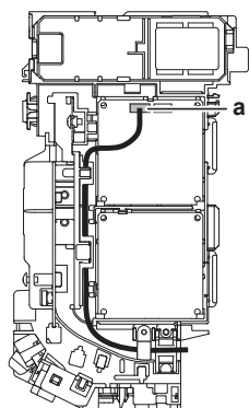
a Ακροδέκτης S21
